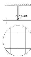
Partial-Plan-Spiegel Ausführung 1
