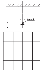
Partial-Plan-Spiegel Ausführung 1
