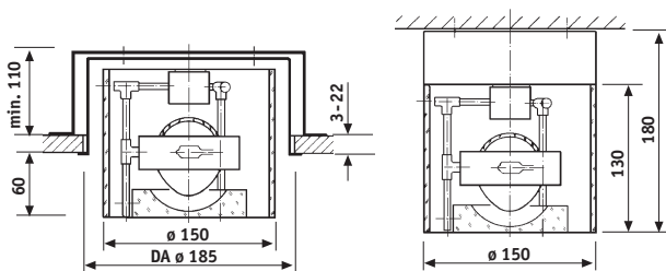
Halbeinbau Typ A1.32.17
