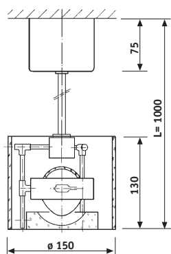
Pendel, incl. ETr. Typ A1.32.19/01-02
